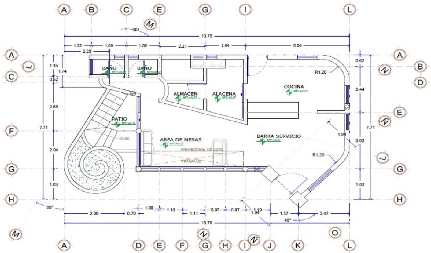
PLANO ARQUITECTONICO PLANTA BAJA ESC:1: 70
