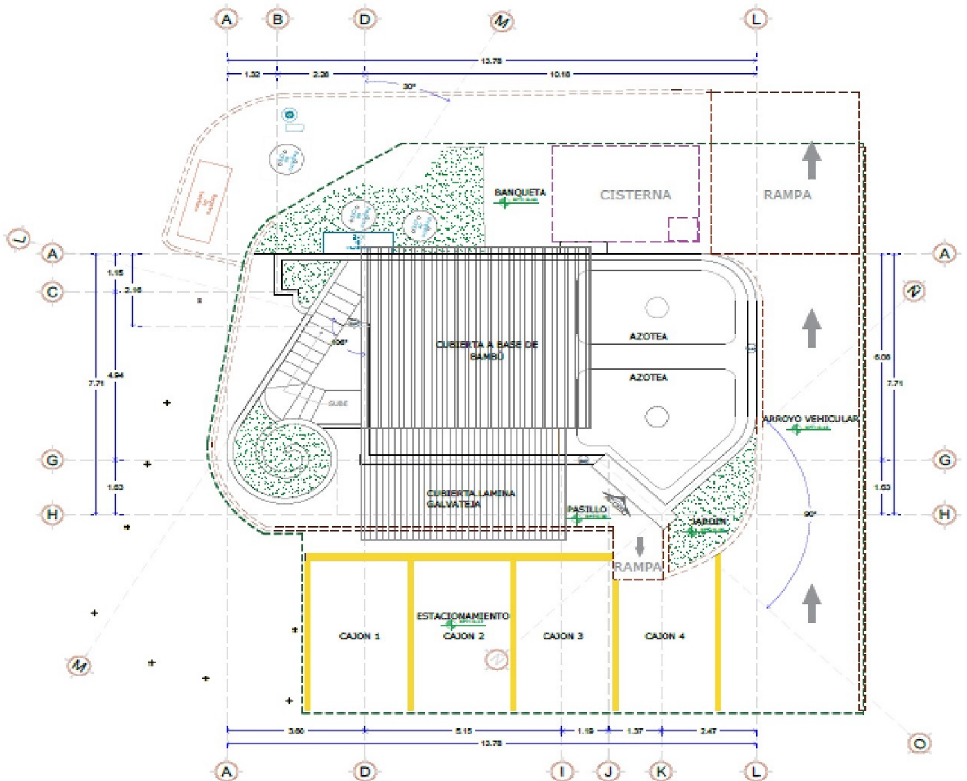
PLANO DE CONJUNTO ESC:1: 70
