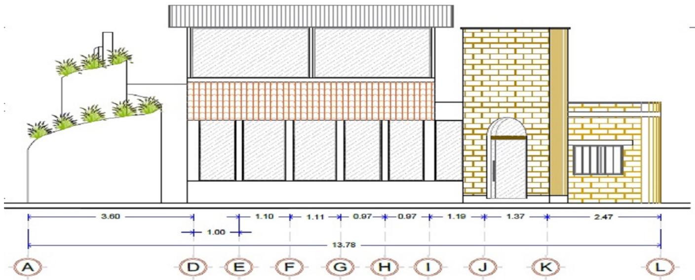
FACHADA PRINCIPAL ESC:1: 70
