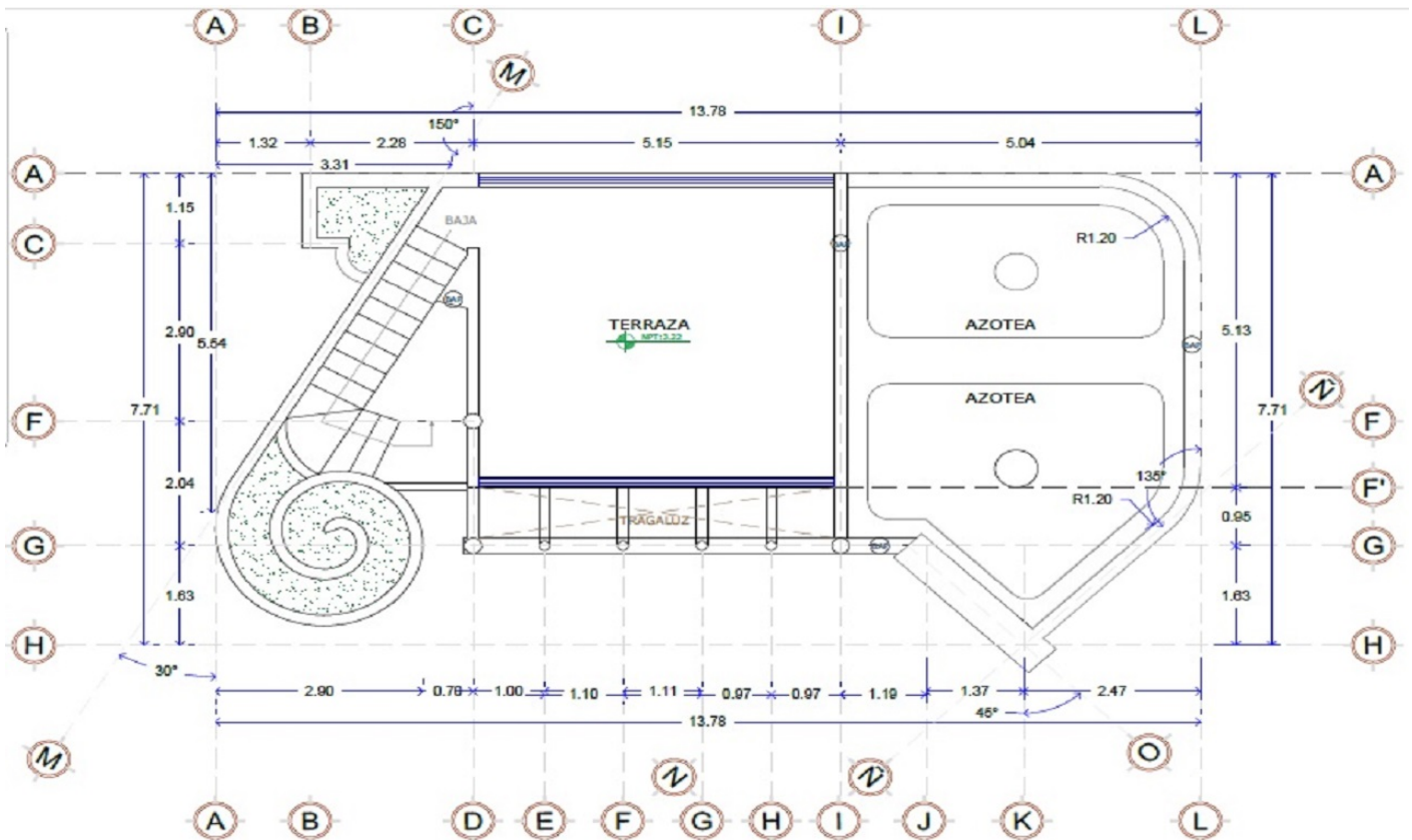
PLANO ARQUITECTONICO PLANTA ALTA ESC:1: 70
