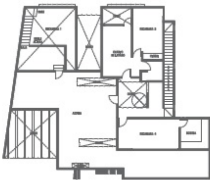
ARQUITECTONICO SEGUNDO NIVEL
